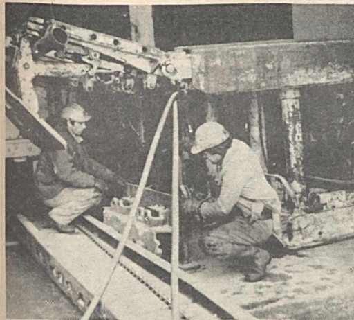
Dowty—Mecsek pajzs külszíni összeszerelése Fotó: Schmidt Zoltán
