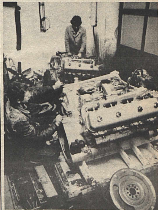
Duga János és Barbarics István autószerelők a Gépkocsi Üzemben egy új KRAZ-teherautómotort tartozékait szerelik fel, a régi motorblokkra az újra.
