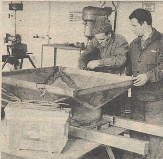
Farkas Sándor és társa újítása a sűrített levegős utárhűtő. A Mecseki Szénbányánál sok csavarkompresszort alkalmaznak külszínen és föld alatt egyaránt. A kompresszor által előállított levegő hőmérséklete sokszor meghaladja a 100 Celsius fokot és emiatt gyakran keletkezik kondenzvíz, ami bejut a működtetett gépbe. Ezt a hibát szünteti meg a Farkas Sándor villamos-csoportvezető által beadott újítás. Nyugati importból eddig is beszerezhető volt ilyen szerkezet, de magas ára miatt és a beszerzési nehézségek miatt csak korlátozott mértékben tudtak ilyen készüléket használni. Fotó: Kórádi Gábor
