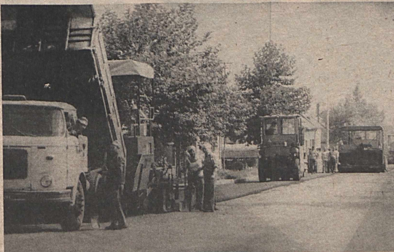
Ütszegélyt építettek, közel 200 víznyelő akna cseréjét végezték el és mintegy 4 kilométer hosszan felújították a pécsi Tolbuhin utat a KEV dolgozói. Fotó: Körödi Gábor
