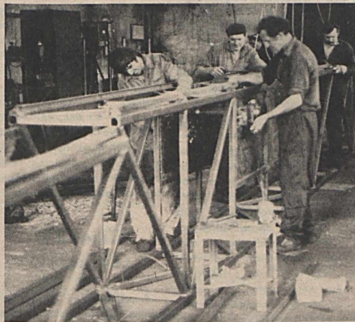
Eredményes tevékenységnek a Mecseki Tanbánya gépészeti szakemberei. Jelenleg — mint képünkön látható — a Somogy megyei Gabonaforgalmi Vállalatnak tároló és forgató berendezést gyártanak.
