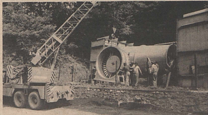
Az Észak-Bányászati Üzem egyes számú főszellőztető berendezésén álló- és forgórészt cseréltek a Központi Gépüzem és a Mecseki Szénbányák Villamos Üzemének szakemberei.
