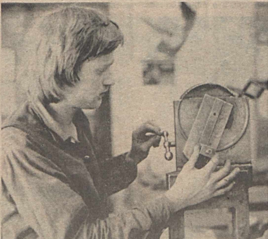
Hogymányos, esztergával gőmböt kialakítani rendkívül nagy feladat. Szendrői Jenő művezető és Hámosi László csoportvezető újítása a képképen látható, gömb esztergálással megkínnyított berendezés. A prototípus az MVE-típusú forgácsológéphez készült. A berendezés segítségével 20–200 mm átmérőjű felületet tudnak megmunkálni. Fotó: Kórádi Gábor
