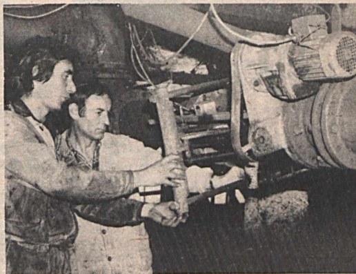
Dávid János lakatos művezető és Szikszai Ferenc villanyszerelő, a Komló Szénelőkesztő Uzem dolgozói adták be újításként a képen látható villanymotor meghajtású elzáró és szabályozó szelepet. A hagyományos megoldásnál egy nyugatnémet szerkezetet használtak, amely kézi meghajtással működött. Az újítással valót és fizikai munkát takarítottak meg. Fotó: Kóródi Gábor
