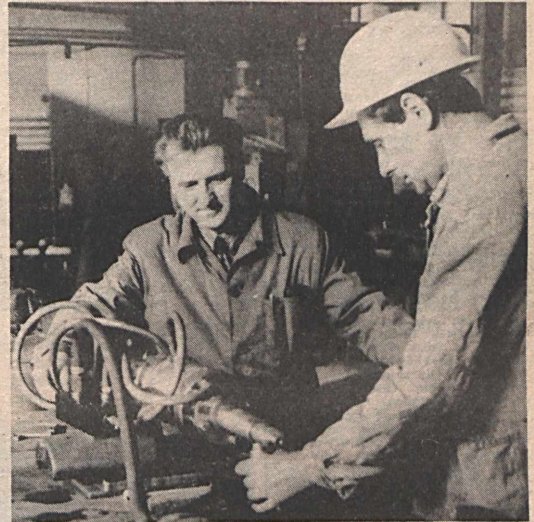
Varga Lajos és Krasz Imre újította a képkünnön látható szivattyút, melyet a bányatüzek oltásánál használnak a habképző puska alapanyaggal való látáshoz. A Mecseki Szénbányánál összesen egy db NSZK gyártmányú szivattyút használtak, ami tőkés importból származott és közel 40 ezer forintba került. A két újító hasonló megoldású berendezést állított elő, melynek paraméterei ugyanolyanok voltak, mint a külföldi gyártmányé. Az új szivattyút hazai alapanyagokból állították elő. Jelenleg kísérletek folynak a szerkezet használhatóságáról. Fotó: Kórádi Gábor
