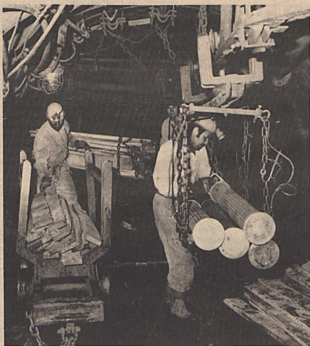
A fejtés anyagellátása a Kossuth-bányauzemnél függőszállító segítségével.
