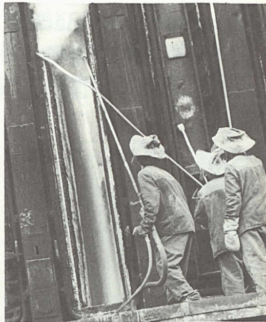
A jelenleg működő két kokszoloblokk egyikén a koksz kitalása után javítják a falazatot
