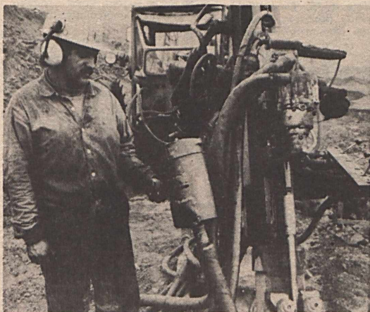
Molnár Imre és Jancsa Demeter, a Kijelölési Uzem dolgozói által megújított Kijelölési Uzemben használatos Böhrer-típusú fűrőklyapácsra szerelhető hangtompító készülék.
