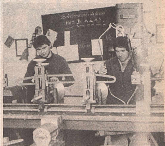
A Mecseki Szénbányák Villamos Üzemének készülő a képpünkön látható tekeresszablon és -formáló berendezés a az újított helyben. A gép elkészítésének ötlete a Mátraaljai Szénbányák Villamos Üzemében született. A szerkezet segítségével sokkal kevesebb tekeressablont kell készíteni. Fotó: Kóródi
