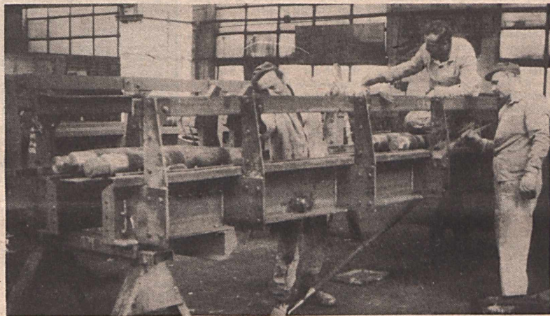
A Központi Gépüzem kézi vezérlésű pneumatikus oknarakodót készít Anna-aknára. A szerkezettel Kossuth-akna 1-es és 2-es pillérjét le tudják fejteti, és a szénkiszárat Anna-akna 3-as szintjéről a társ szintre lehet hozni. A Központi Gépüzem rendkívül gyorsasággal készítette el a vasszerkezeteket, aknaoklakokat, aknaelzáró-ajtókat, a ki- és betoásoldali lengőpadokat és a vasszerkezeteket. Képünkön két darab adagoló vágóábrát utolsó munkafolyamatait végzi a festőbrigád. A gyors ütemű gyártással egy időben a munkaszüneti napokon a szerkezet beszerelését is folyamatosan végzik a gépüzem szakemberei. Fotó: Kóródi
