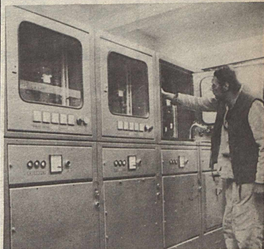
Boszó Sándor a K IV-es aknán a 6-KV-os kapcsoló berendezést ellenőrzi
