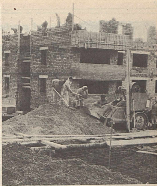
Bányák miatt jelentős számú lakóházat kell szanálni a közeljövőben Komlón. A Mecseki Szénbányák a kieső lakásszám pótlására Szilvásbán a viztorony környékén a VI. ötéves tervben hét, egyenként 16 lakásos épületet épít. Az első épületet decemberben már át is adták, jelenleg a második ház kivitelezésén dolgozik a Karbantartó Üzem. Fotó: Kóródi
