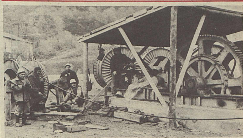
Az V. ötéves terv legnagyobb beruházása a Mecsekben a Kossuth IV-es akna építése. Még a hetvenes évek végén kezdték el a mélyítést az Aknamélyítő Vállalat szakemberei, de a teljes átadása csak a VI. ötéves tervben valósul meg. Az új létesítmény átadására a közeljövőben kerül sor. Képünkön: a Villamos Üzem szakemberei az elektromos kábelek beépítését végzik. (Képröportunk a 7. oldalon).
