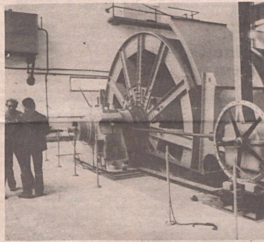
Az Országos Bányagépgyártó Vállalat készítette a BATI tervei alapján a kétdobos szállítógépet
