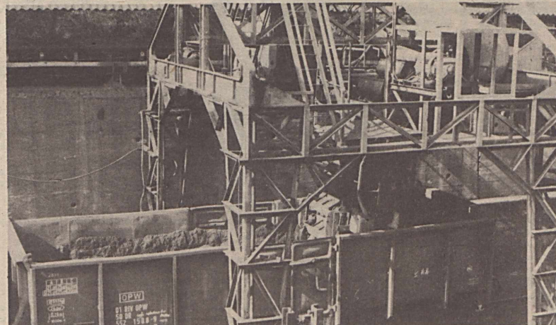
A Nagymányoki Brikettüzemben az elmúlt években sok, a nehéz fizikai munkát megkönnyítő gépet állítottak termelésbe. A képen látható berendezés automatikus, óránként 40-50 tonna szenet tud kirakni a vagonokból. Foto: Kóródi Gábor
