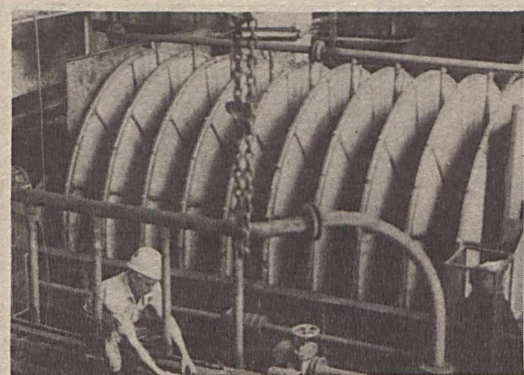
A széniszap víztelenítésének a legkorszerűbb eljárással történő technológiai berendezése látható a képen. A társak 100 négyzetméter felületű szűrőkkel rendelkeznek. Kép: Kórodi Gábor
