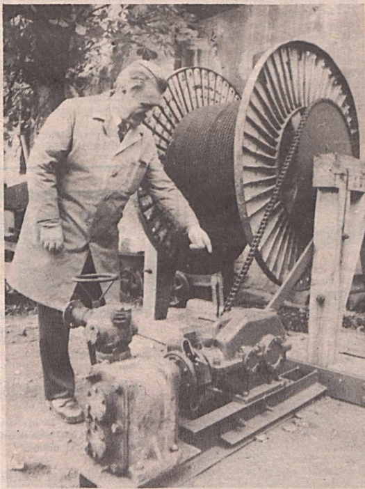
Kötél- és kábelcsévlő berendezést készített Vasasbányán Varga Lajos és Keszericze Rudolf. Az újításként elfogadott berendezés a nehéz fizikai munkát könnyítette meg. A csévlőt külszínen és a bányában egyaránt használhatják, mert a gép sürített levegő-meghajtással működik. Fotó: Kóródi
