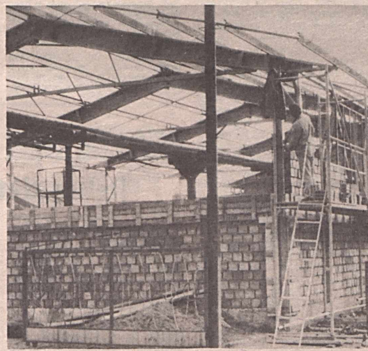
Cseregépártól épít a Mecseki Szénbányák Karbantartó Üzeme Komlón a Központi Gépüzem udvarán. A helyiségekben tárolják majd a megjavított gépeket és ugyanitt kap helyet az anyagmozgatásnál nélkülözhetetlen targoncák. A létesítményt a gépüzem saját beruházásából valósítja meg. Az épületet még idén szeretnék átadni.
