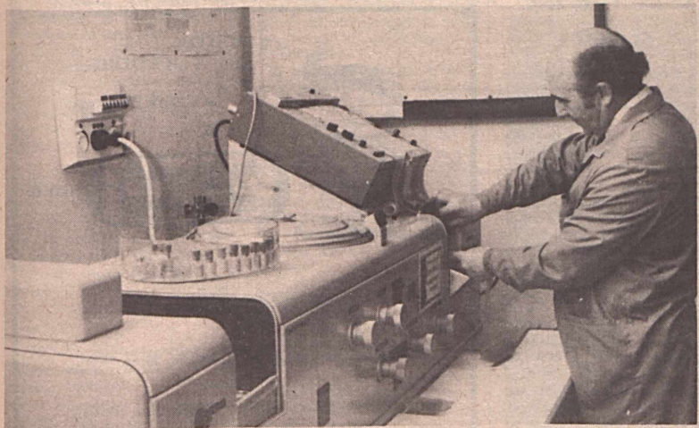
A Mecseki Szénbányák Kutatási Üzemében Czihai Ferenc okleveles kutató vegyész-mérnök, egy infravörös spektrálfotóméteren a szénpor összetételét vizsgálja.
