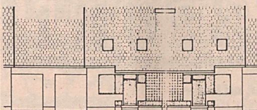
UTCA FELŐLI HOMLOKZAT M=1:100
