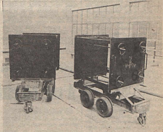
Több éves gondot oldott meg Podpácz László és szocialista brigádja a zótkai bányánál állomást dolgozó, a képen látható gyorsjáró ajtó elkészítésével. A robbanásálló kivitelben készült és falozott tüdőgátba építhető szerkezet biztosítja a robbanásálló előgátok biztonságos és gyors zárást. Foto: Nemesi Árpád
