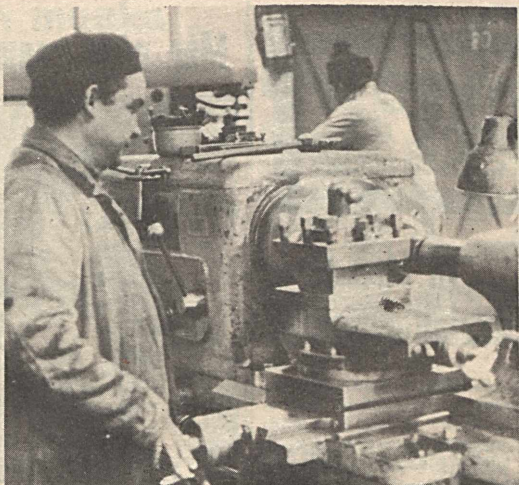
A nagy értékű gépekhez, berendezésekhez egyik-másik alkotórész a széntermelő üzemek javító műhelyeiben állítják elő. Képünkön Gadó Géza esztergályos Beta-bányán, aki nemrégiben kapta meg a Kiváló Dolgozó kitüntetést, az SL-E típusú fúrógéphez a vezetőhüvelyt esztergálja. A szerkezetet a széntelepek nagy átmérőjű átfúrásánál használják. Fotó: Kóródi Gábor
