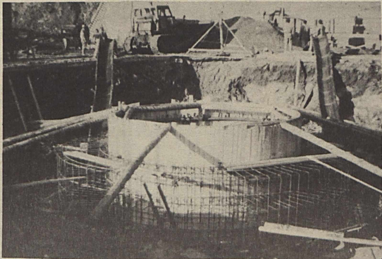
Utolsó fázisához érkezett a komlói aknamélyítők munkája a K—IV-es aknán. Most már az aknafej kidolgozásán tevékenykednek, amelyhez 2800 köbméter anyagot mozgattak meg.
