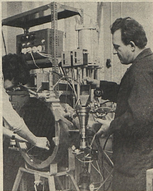
Uzembe helyezték a Mecseki Szénbányák kutatási műhelyében az új, nagy teljesítményű robbantókamerát. A berendezés segítségével sokkal több kísérleti robbantást tudnak végrehozni. A mért eredmények a nemzetközi szabványoknak megfelelnek. Képfőnök a kísérleti kamrában elhelyezik a szénpor robbanásához szükséges alapanyagokat. Fotó: Kóródi Gábor
