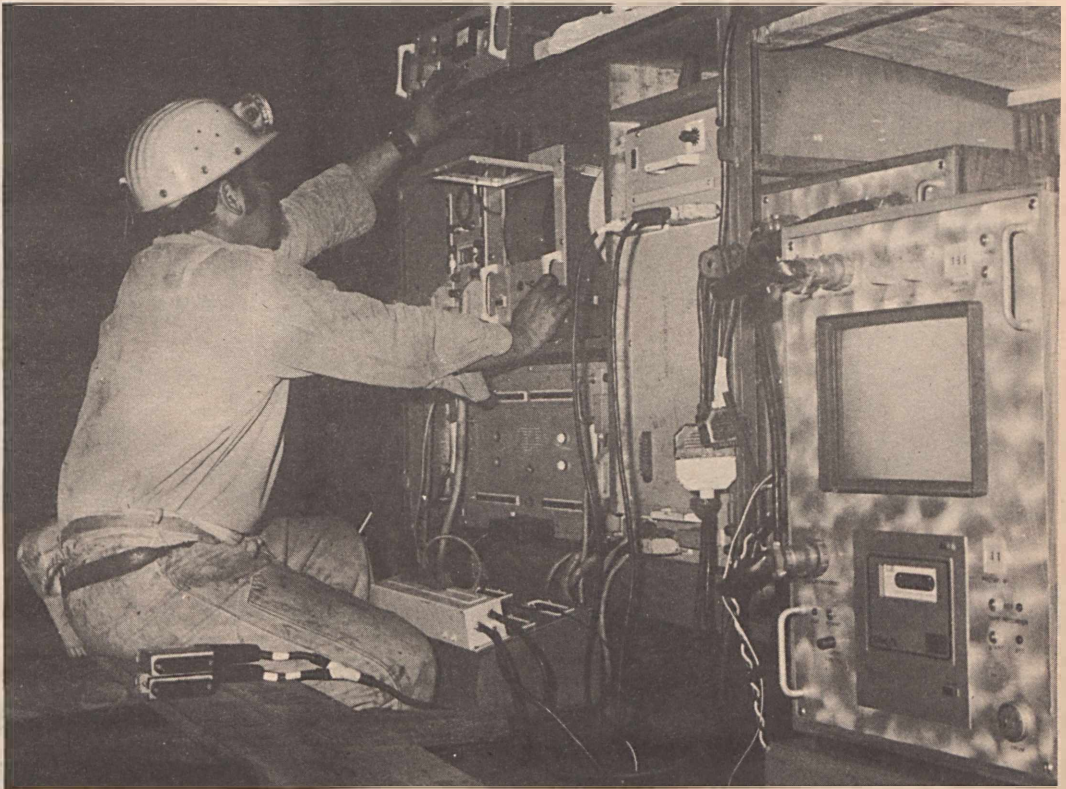
A kísérleti nagyfrekvenciás, tv-képernyős, szeizmikus mérőműszer munka közben, Vasasbányán
