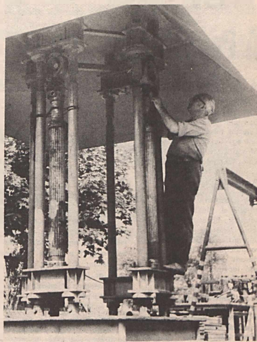
A kutatóintézet által kifejlesztett könnyűfém-támok a mérpadon
