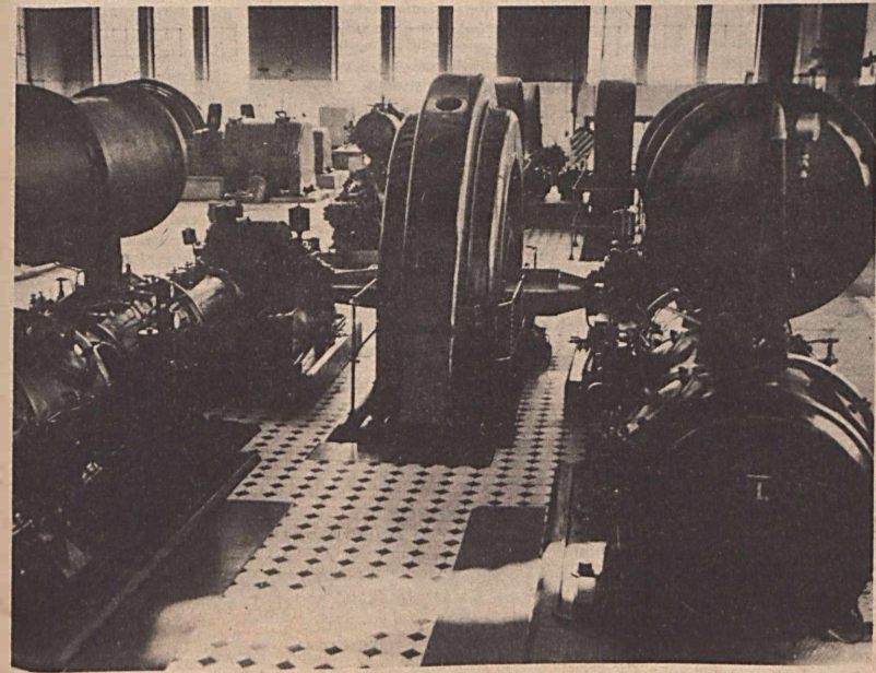
Az István-aknán működő turbógépház, amely a bányá sűrített levegő ellátását biztosítja
