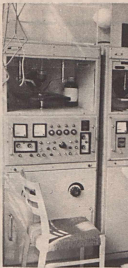
Ezekkel a műszerekkel azt vizsgálják, milyen a szigetelések biztonsága
