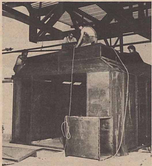
A fényezőműhely szűrítőkameráját szerelik össze
