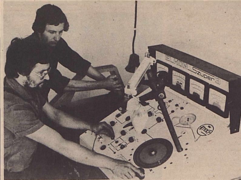
A próbapadon érzékelőket és elektronikus gépjelző-alkatrészeket tudnak beállítani
