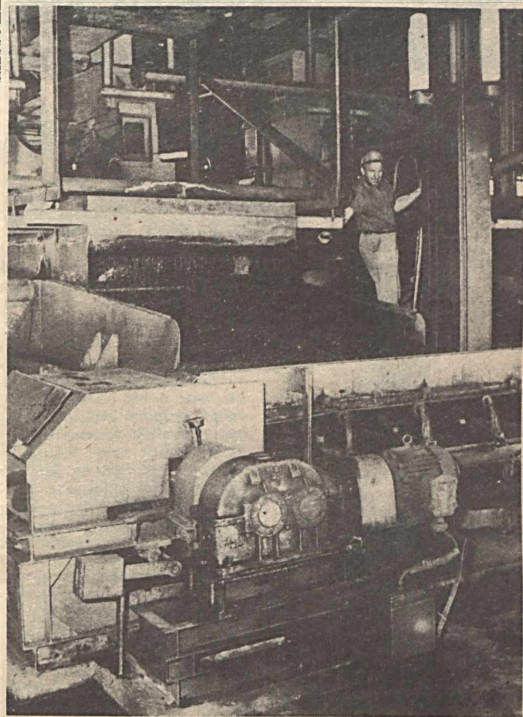
A minőségi szén előállítását szolgáló szitator a Pécsi Szénelőkészítő Üzemben. (A két szénelőkészítő Üzem termeléséről tudósítás a 3. oldalon.)
