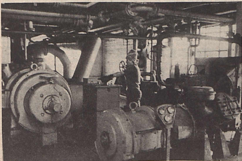
A Komló Szénelőkészítő Üzem komp kompresszorai — működés közben
