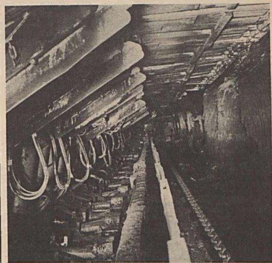
Teljesen gépesített fejtés
