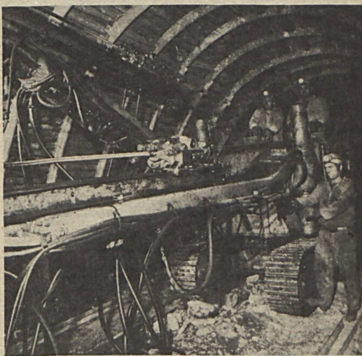
A Tamrock fúrókocsi megkíméli az izületet
