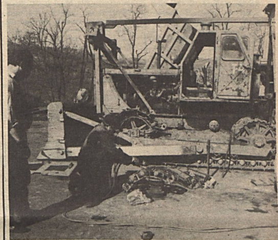
T 4-es tológép lánctalpát javítja Juhász Gyula hegesztő és Bischof János szerelő.
