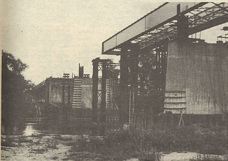
A csengeri híd acélszerkezete a hidpillérekre húzás pillanatában Jakab József felv.
