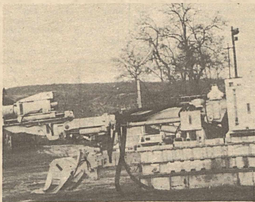
Vasas-bányán nemsokára üzembehelyezik az Impact Ripper vágathajtó gépsort. Képünkön a berendezés — még a külszinen. Fotó: Tomasek Lajos
