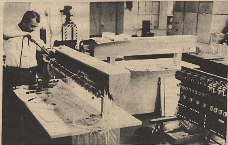
A Villamos Üzem — a Mecseki Szénbányák üzemai részére végzett szolgáltatások mellett — számos jelentős munkát készít idegen vállalatok megrendelésére is. Képviselet: műszerasztal szerelése a pécsi „Zipernovszky Károly” Gépipari Technikum számára. Az üzem újhegyi (köz-ponti) műhelye az iskolának egy teljes próbatemet állít össze villamosmotorok, generátorok és dinamók működtetésének tanulmányozására. Kóródi Gábor felvétele
