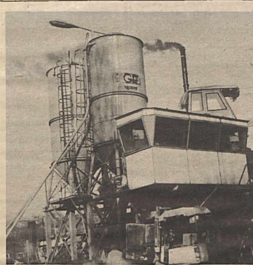
Beton- és Vasbetonipari Művek komlóji telepén új gyártó sort építenek. Amíg a rekonstrukció elkészül, ideiglenes, C-16 típusú betonkeverőt (képünk) állítottak üzembe, hogy folyamatos legyen a munka.
