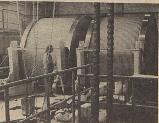
A szállító gép óriás dobjai — még kötél nélkül.
