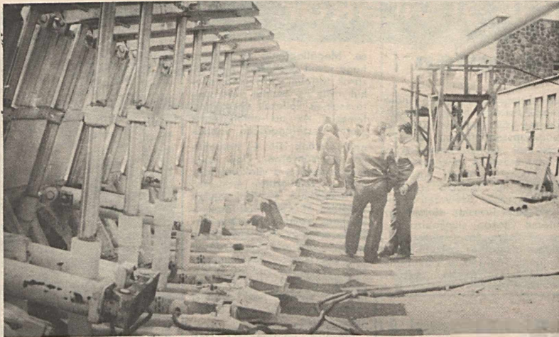
Béta-bányán az ASCS komplex berendezés szerelési munkálatait végzik
