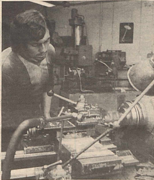
Kovács Ottó (MOM komlói gyáregysége) olajfékhengert készít
