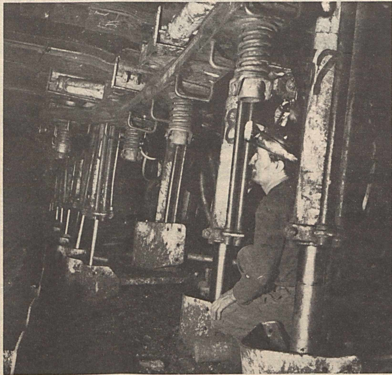
Az István-aknán beépítésre tervezett lengyel SOW-40-es meredek telepi fejtesbiztosító berendezés, ez alkalommal még Alsó-Sziléziában.
