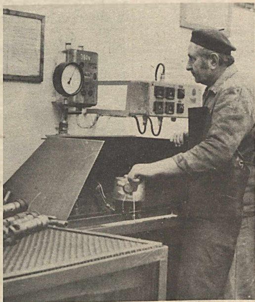
A német „Tyssen” hidraulikus bányatámok vezérlőszelvények beállítását végzi Bori István, a Központi Gépüzemben.
