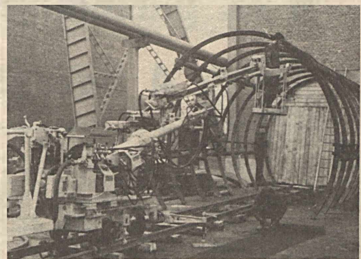
Vállalatunk 2 db BUR—2B típusú fúrókocsit szerzett be. Képvén a Zobák-bányai gép látható külszíni próbajáratáson (Fotó: Gutt)
