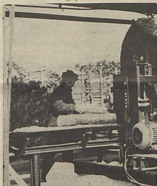
Szutor Sándor, a Dózsa György szocialista brigád tagja „Ezresz” szalagfűrészgéppel negyedeli a farönköket a Központi Anyagellátó Üzemben. Maletics László felv.
