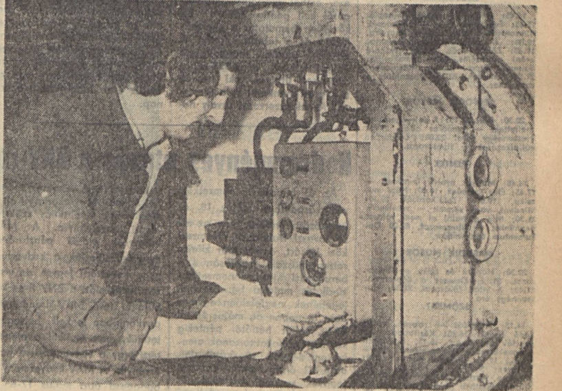
Schaller Róbert a központi műhelyben egy IT-3 SA 2000 klívoltamperes, bányában használatos lengyel gyártmányú transzformátor szerelését végzi.
