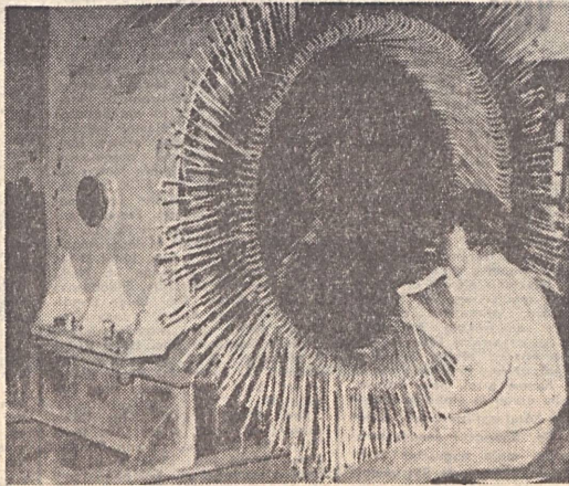
A Villamos Üzem legjellemzőbb munkái közé tartozik a villamos motorok felújítása. Képközpön: a Ward—Leonard állórész tekerése.
