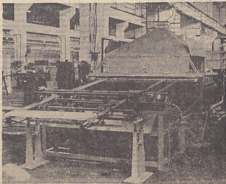
A képen a Központi Gépüzem által — az Egyesült Ízzó megrendelése alapján — gyártott ZFL 28-05 fénycsőbeégető berendezése látható, amit Irakba szállítanak. A rendkívül nagy pontosságot igénylő gép elkészítésével az üzem dolgozói jól vizsgáltak. A közeljövőben még tíz gép sor elkészítésére kerül sor. Foto: Nemesi
