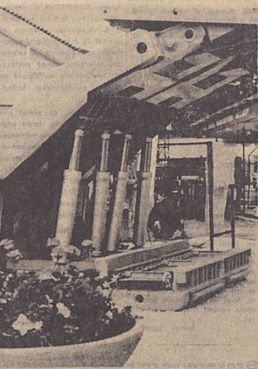
A Kossuth-bányán is alkalmazott páncélpajzs a 7-es pavilonban.
