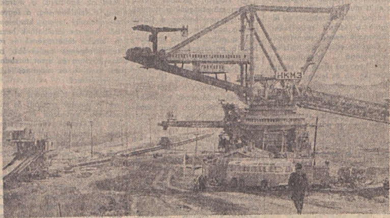
A Novokramatorszkban készült maratórész exkavátor az „Aleksandrijaugol” kombinát felszíni fejtésén dolgozik
