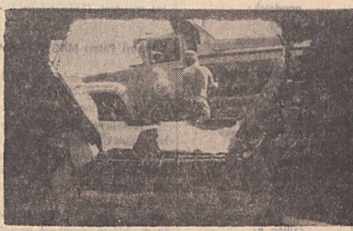
Széchenyi-aknában a tehérgépkocsiról a buktatóba ömlő szénoszta-lyozó-rácson keresztül kerül a szállítószalagra. A képen: a buktató előtt áll a tehérgépkocsi.
