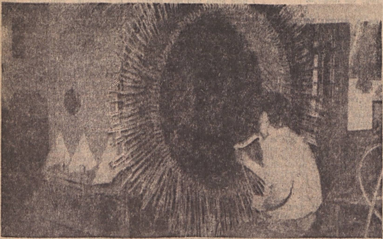
A tekerész műhelyben egy Ward Leonard féle állórész tekerésében folyik. (Foto: B. Anna Teréz)
