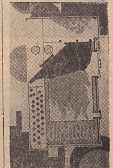
A „Mecsek 15” kiskazán belső szerkezetének keresztmetszete.
