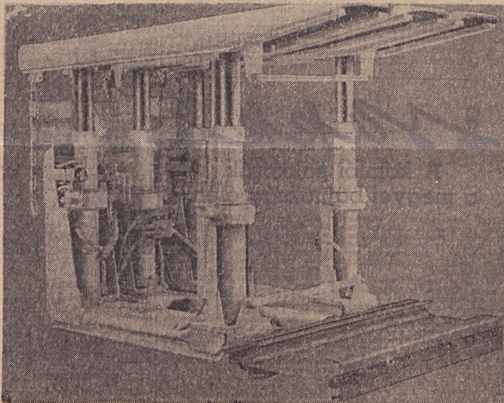
A három angol cég gyártmányai közül képünkön a 3 keretes, 6 támas „Dowty” biztosító-berendezést mutatjuk be.
