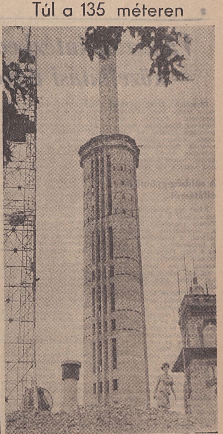
Jó ütemben halad a Misina-tetői tv adótorony építése. Az építők július 26-án elérték a 135. métert. A torony átmérője itt öt méter. Innen viszont már csak három méteres átmérővel haladnak tovább újabb 37 métert. A torony építését szeptemberre befejezi a Baranya megyei Állami Építőipari Vállalat. A belső szerelés mintegy másfél évig tart majd, s az új adó várható üzembehelyezésére 1970-ben kerül sor. (Császár Zoltán felvétele)
