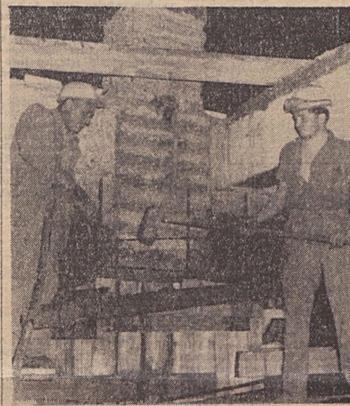
Toncz Henrik kőműves brigádvezető és Lutz János kőműves betonnal tölti ki a zsalu és az oszlop közötti réteget. A vasbetonkoszorú megerősíti a tartóoszlopokat, így azok alkalmasak lesznek a később beszerelendő súlyos gépek tartására.
