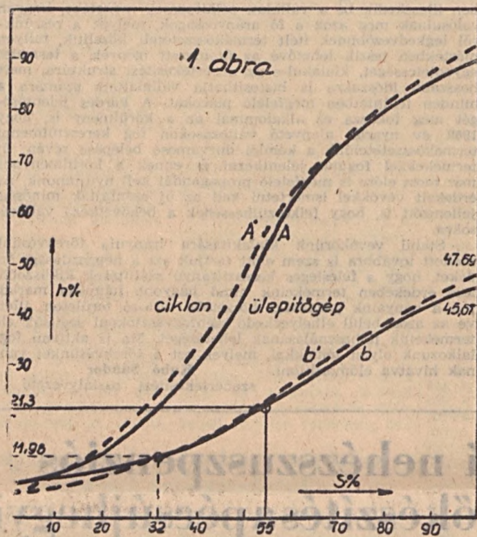
Az ülepitőgépre és a ciklonra feladott nyersaprószén mosási görbéi
