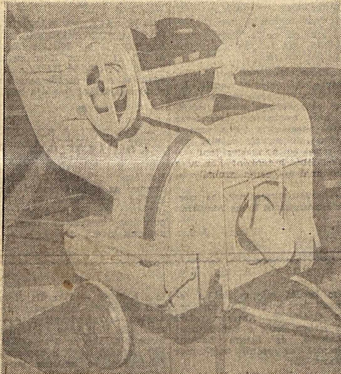
Sokan megcsodálták a Prantner Ferenc által készített ferde-dobos betonkeverőt, amely hű mása az eredetinek
