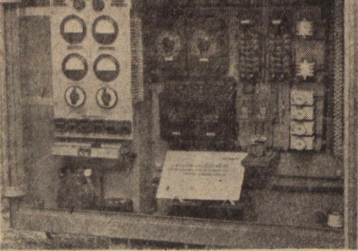
APSPa 100 a típusú önműködő mozgó egyenirányító állomás, a kiállítás egyik érdekes darabja.
