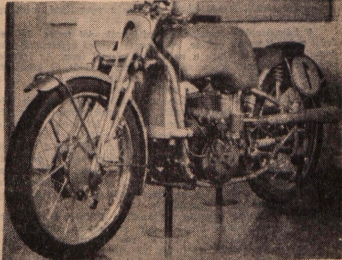
Az 500 köbcentiméteres, 40 lóerős, kétittemű vízhűtéses DKW 1937-ben volt szűr
