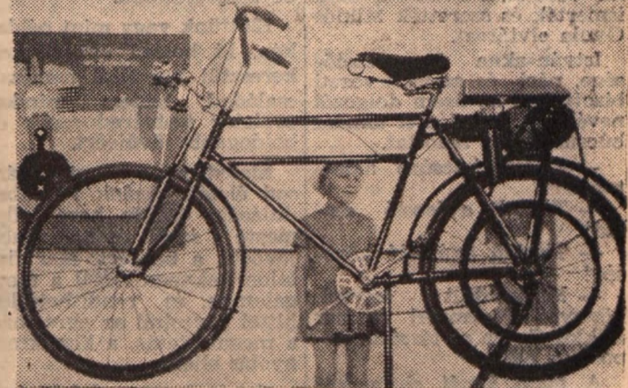
A kerékpár „dongó” segédmotorok őse az 1921-ben gyártott 122 köbcentiméteres, egy lóerős DKW
