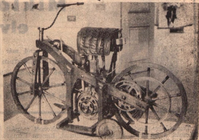
1885-ből származik a motorkerékpár őse, az 58 köbcentiméteres petróleum üzemanyagú, egy hengeres, négytémű Daimler. A fákereket szíjjátételes fogaskerekek hajtják.
