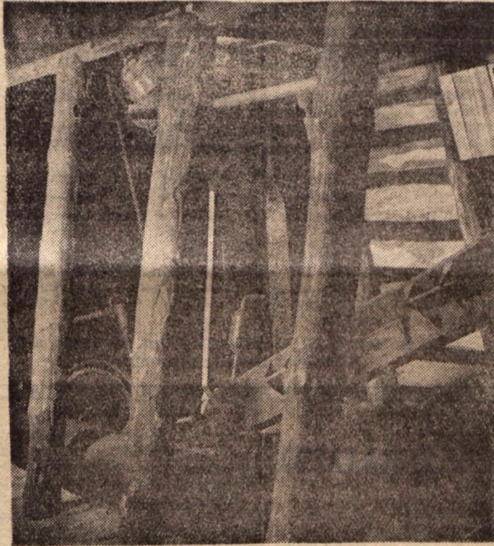
A földszinti 2. számú gépkamrában látható a Kista-féle földrakóval szénben végzett elővájás
