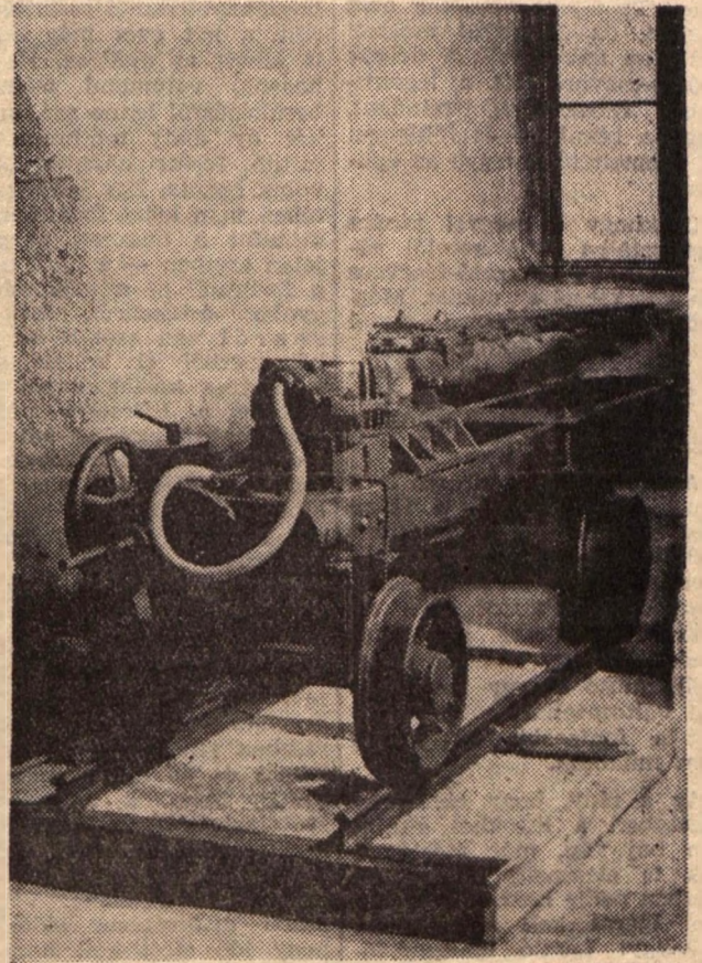
A múzeumban kiállított Korffmann-féle réselőgép eredeti je
