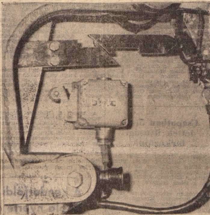
A kép felső részén jól látható a biztonsági retesz. Ha a kampók összeakadnak, a gépész nem indíthatja meg a kast. A jelzés hatására viszont egy mágnes magához rántja a felső kampót, ez által az indítóör rúdja szabaddá válik, a dob megindul, a kas mozgásba jön.
