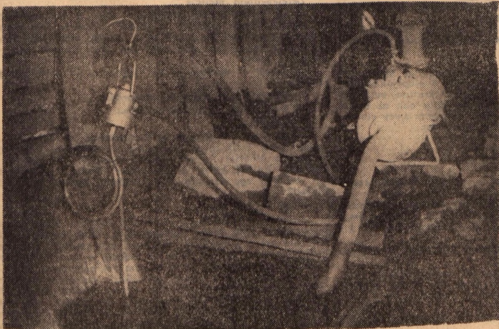
A pneumatikus szivattyú-automata üzem közben Zobák-akna I. szintjén
