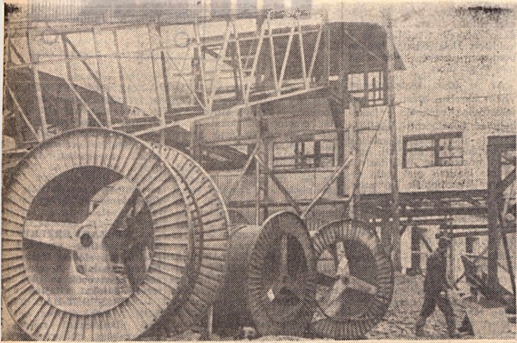
Az Északi Bányászati Üzem rekonstrukciója folytán szükségessé vált a régi szénosztályozó lebontása és egy újnak a felépítése. Az új szénosztályozó építése már megkezdődött, s a tervek szerint ez évben befejezést is nyer. A munkálatokat Kossuth-bánya, a Villamos Üzem és az Északi Üzem közösen végzi. Felvételi az építés alatt álló szénosztályozót mutatja.
