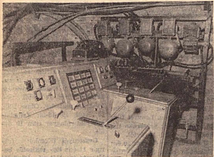
A sok millió forint értékű tervezőmunka egyik megtestesülése látható a képen. Nemesi Árpád felvétele a korszerű Bata-aknai csatlózpultot örökítette meg. Háttérben a régi jelzőberendezés látható, amelyet azóta már leszereltek.
