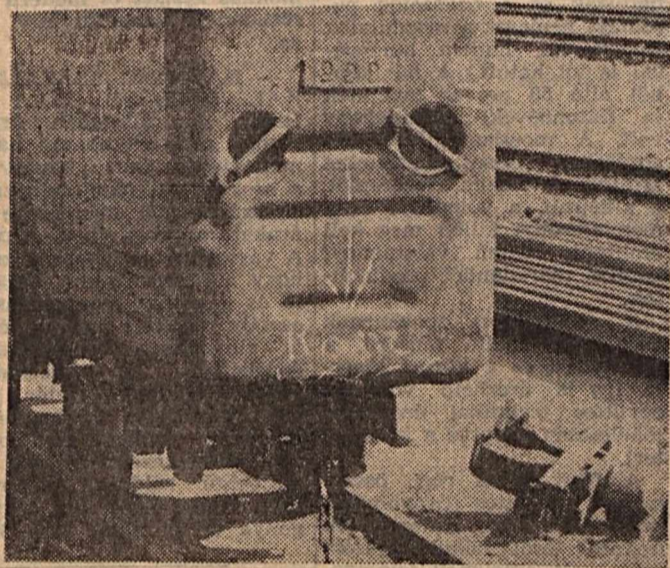
A rossz csille, amely halálos áldozatot követelt. A felvételen is látható, hogy a csille ütközője hiányzik. A vizsgálat idejére előkerült vonószerkezet a kép jobb sarkában.
